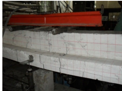
Gambar 10 Pola retak balok kontrol (BK).
