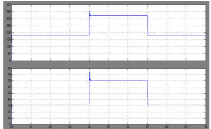
Gambar 21 Arus Sisi Primer dan Sekunder Kondisi Gangguan Luar.
