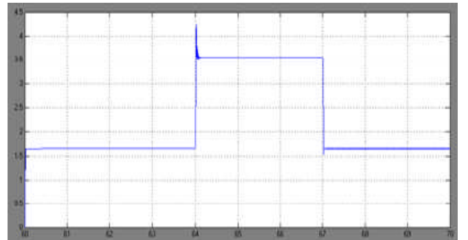
Gambar 23 Arus Kerja Diferensial Sisi Sekunder Kondisi Gangguan Luar.
