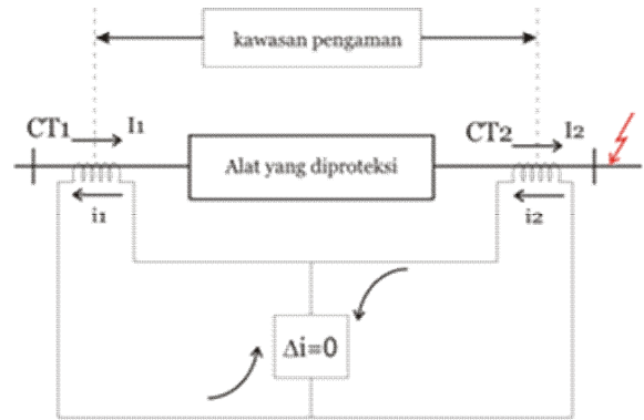
Gambar 4 Kondisi Gangguan Luar Rele Diferensial.
