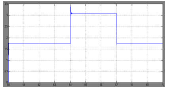
Gambar 22 Arus Kerja Diferensial Sisi Primer Kondisi Gangguan Luar.
