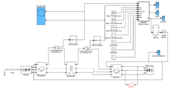
Gambar 20 Simulasi Kondisi Gangguan Hubung Singkat di Luar Daerah Pengamanannya.
