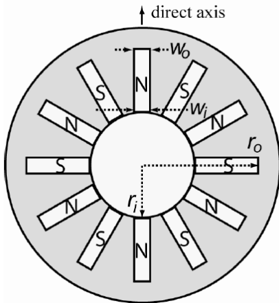
Gambar 13. Skema rotor
