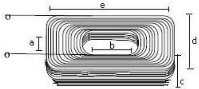
Gambar 14. Kumbaran 3 dimensi
