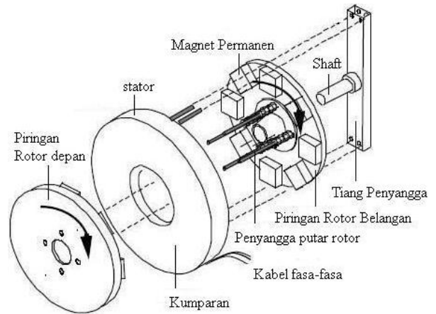
Gambar 9. Konstruksi generator
