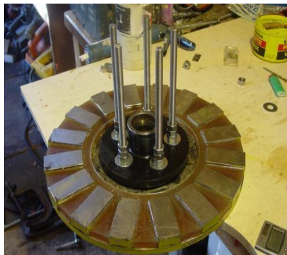
Gambar 1. Susunan magnet permanen pada piringan rotor
