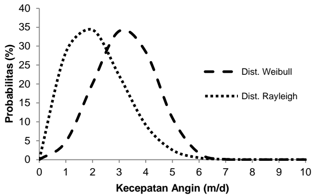
Gambar 5. Distribusi Weibull dan Rayleigh untuk Peisir Cilacap
